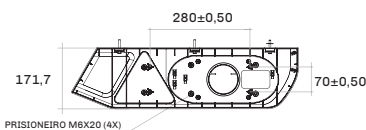
Fixação traseira
