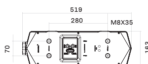
Fixação traseira
