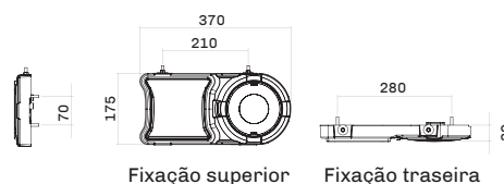
Fixação superior
